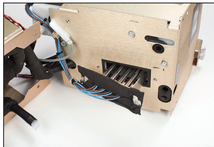
Obr. 8-50 Demontáž ohříváče (krok 4)
