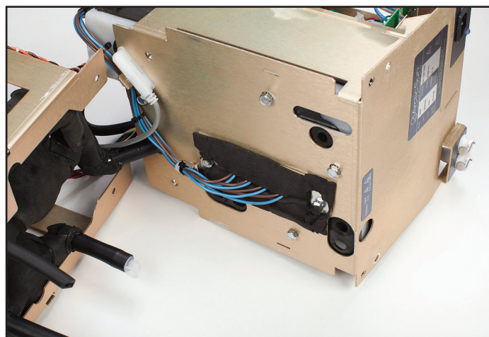
Obr. 8-49 Nádrž a ohříváč s označenými kabelovými svazky, které mají být odstraněny (krok 2)
