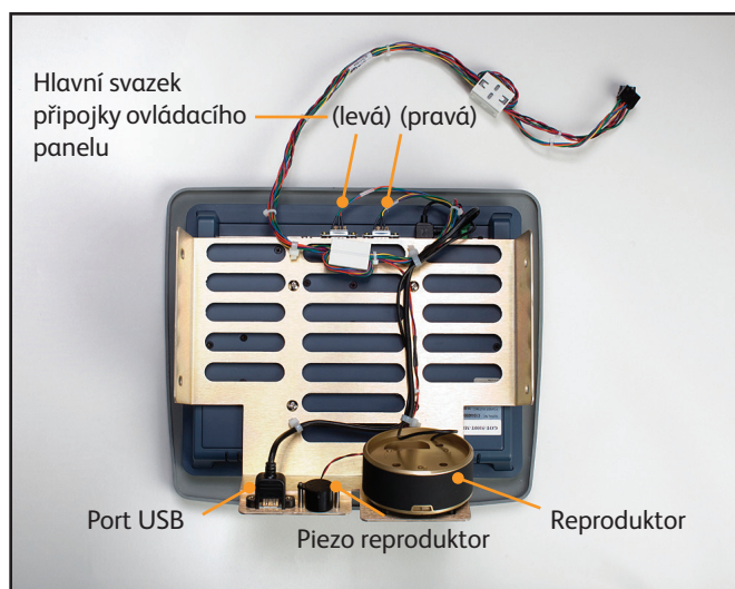
Obr. 8-55 Ovládací panel (pohled zezadu)
