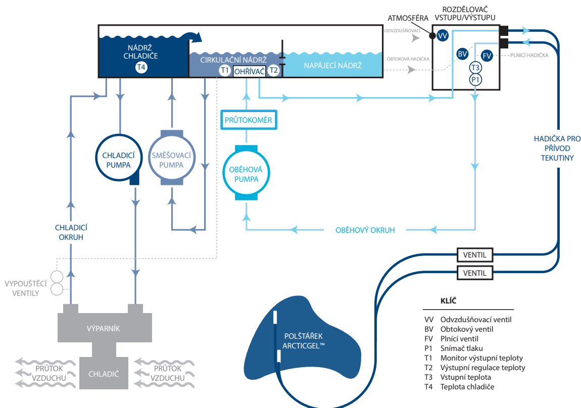
Obr. 2-1 Hydraulické schéma
