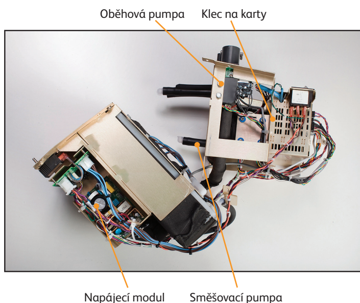
Obr. 8-26 Vnitřní součásti rozdělené na dvě části (2 pohledy)
